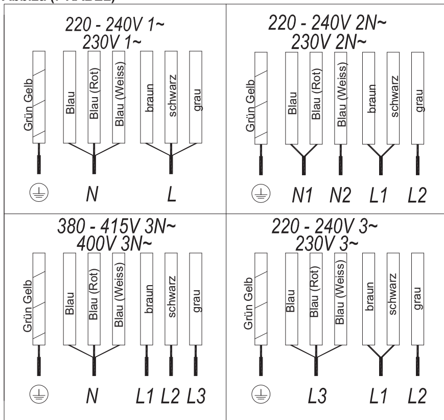
Abb.2a (7 KABEL)
