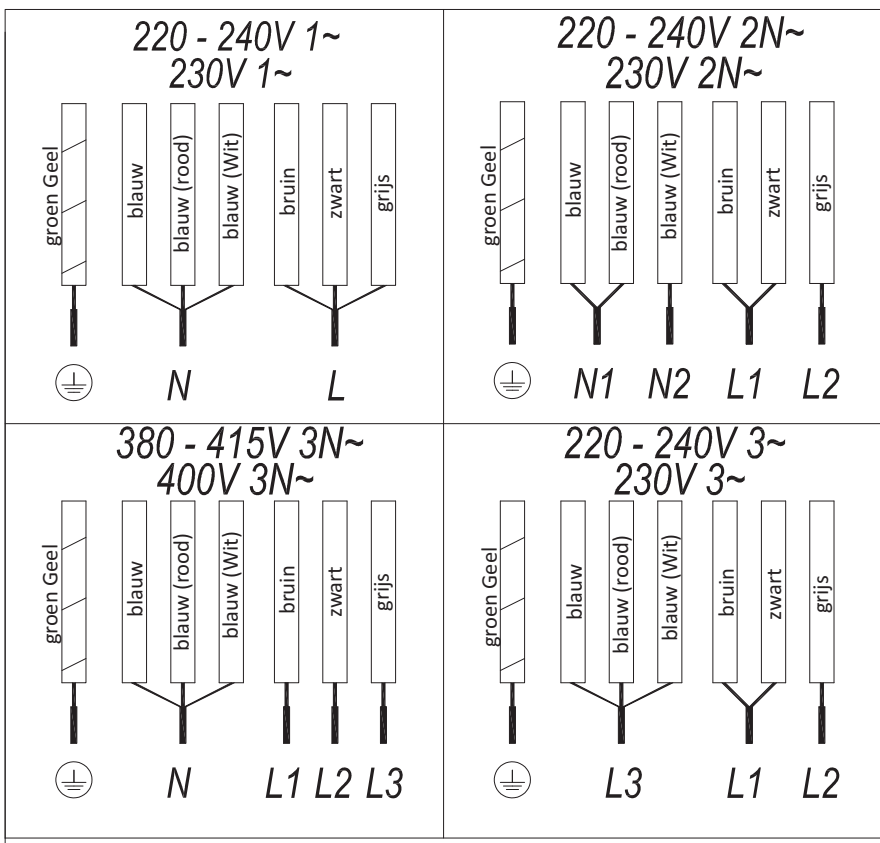
Afb. 2b (7 DRADEN)
