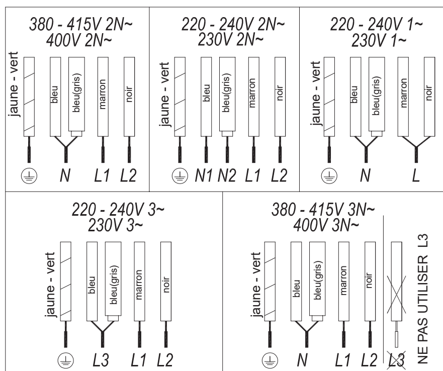
Fig.2a (5 FILS)
