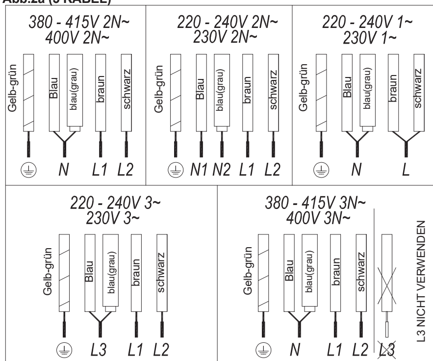
Abb.2a (5 KABEL)
