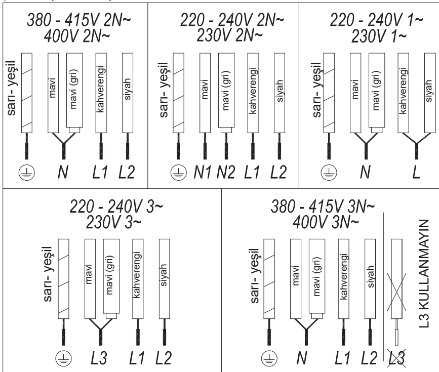
Şekil 2a (5 KABLO)
