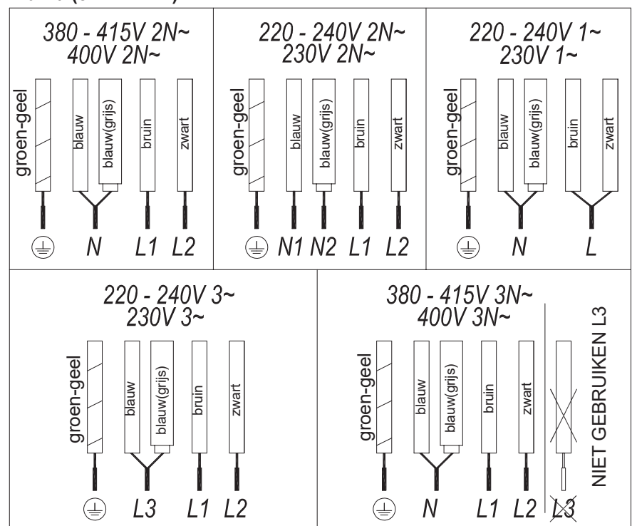
Afb. 2a (5 DRADEN)
