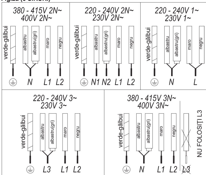
Fig.2a (5 SIRURI)
