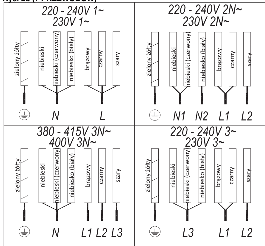
Rys. 2b (7 PRZEWODÓW)
