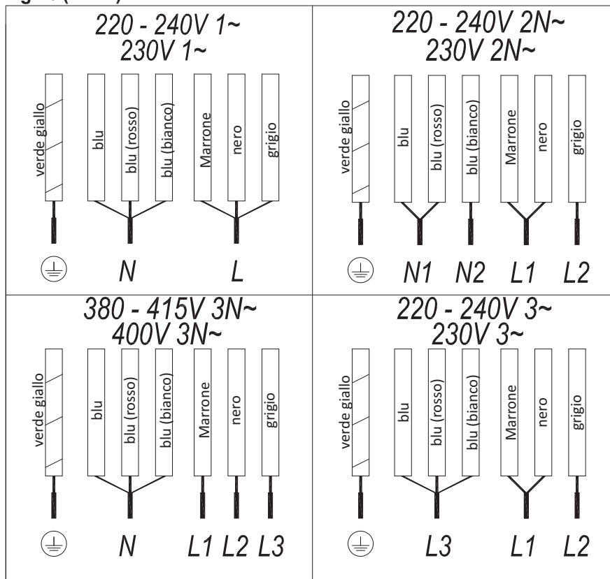
Fig.2b (7 FILI)
